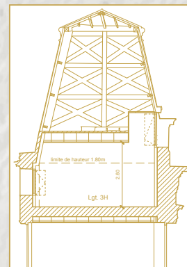
Plan de coupe 3H
