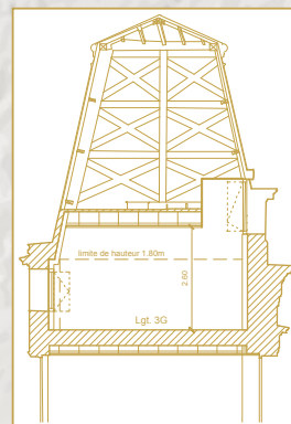
Plan de coupe 3G
