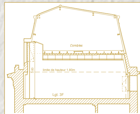
Plan de coupe 3F
